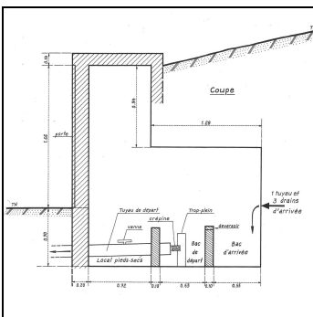
Coupe d'un captage par drain
